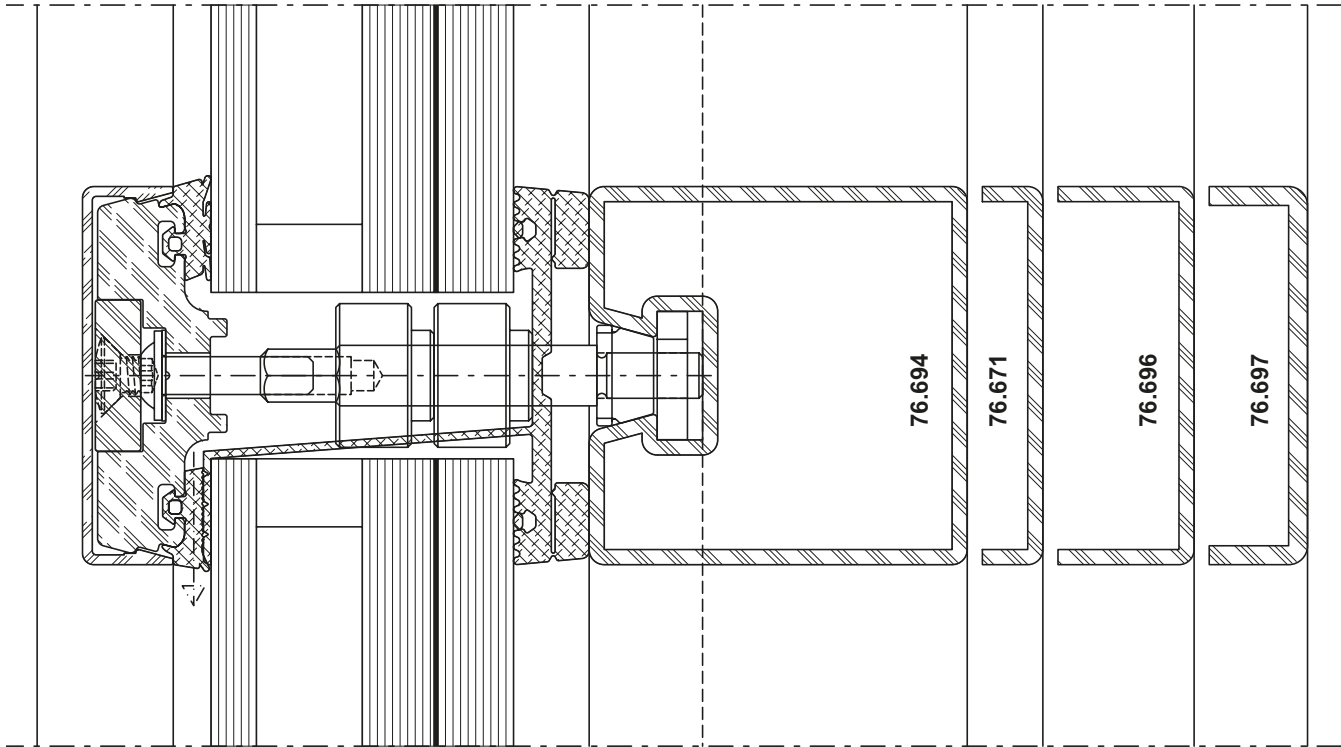
VISS Fassade Riegel-Detail Ansichtsbreite 50 mm
